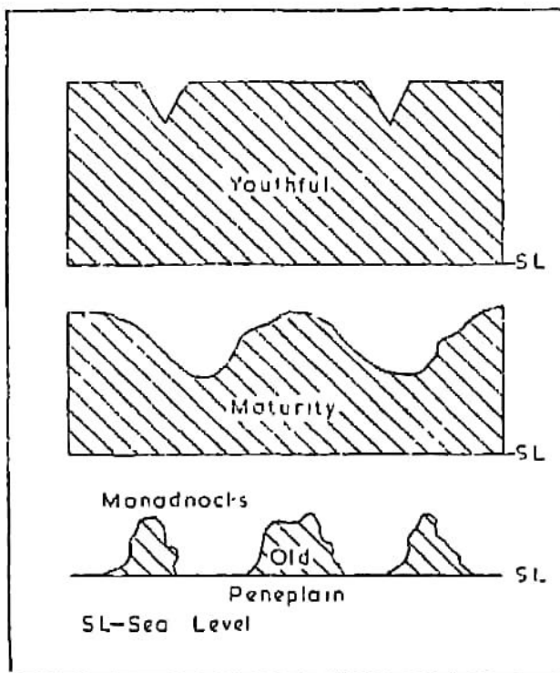
Fig. 28. Fluvial Cycle
