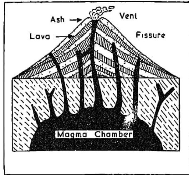
Fig. 53. Volcano
