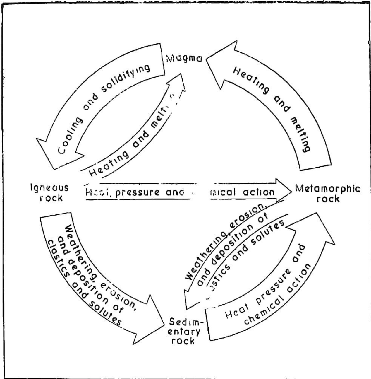
Fig. 18. Rock Cycle
