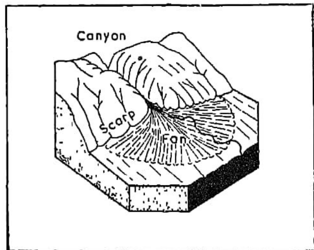
Fig. 33. Alluvial Fan
