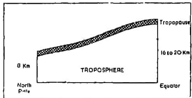
Fig. 57. Troposphere
