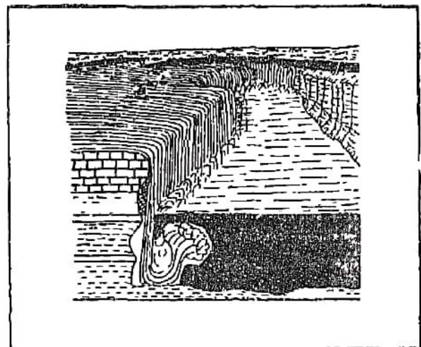
Fig. 29. Niagara Fall
